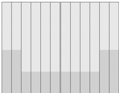
X088 - Culla - Base totale mm 580 x h. centrale mm 99,5 - Lato superiore mm 89 x h. esterna mm 186,5
